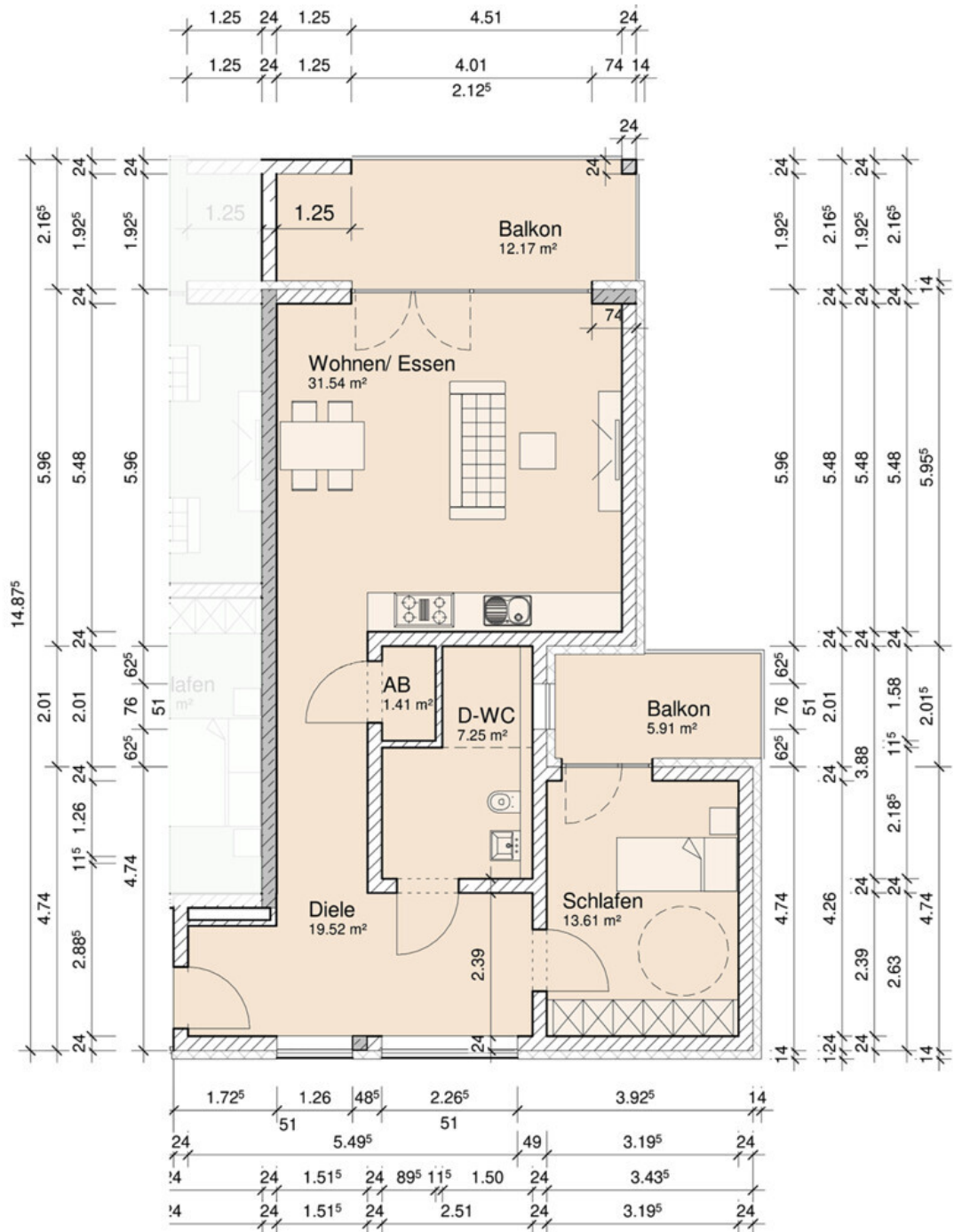
Luma Grundriss Wohnung 4 bemaßt
