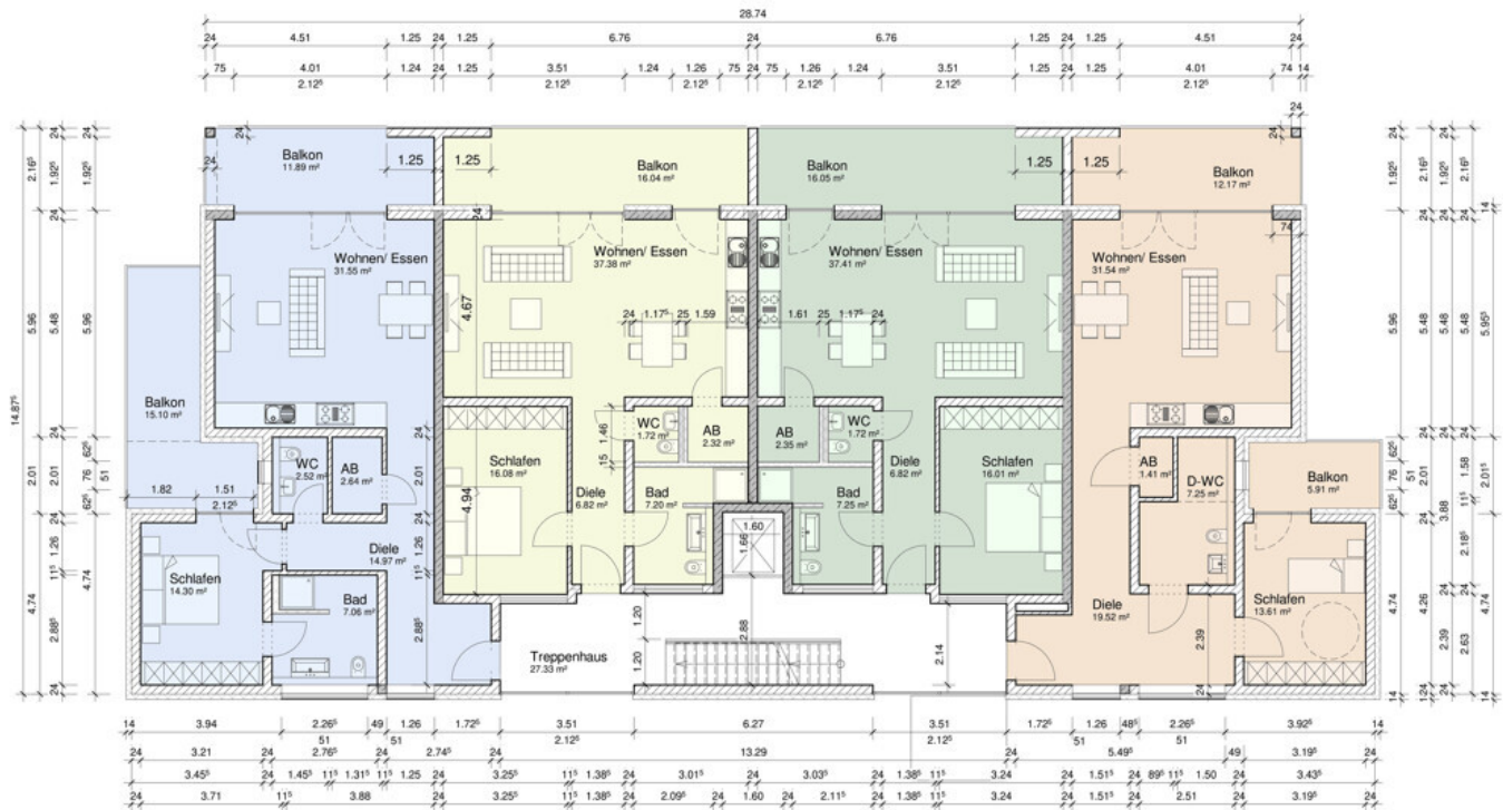
Grundriss 1. Obergeschoss
