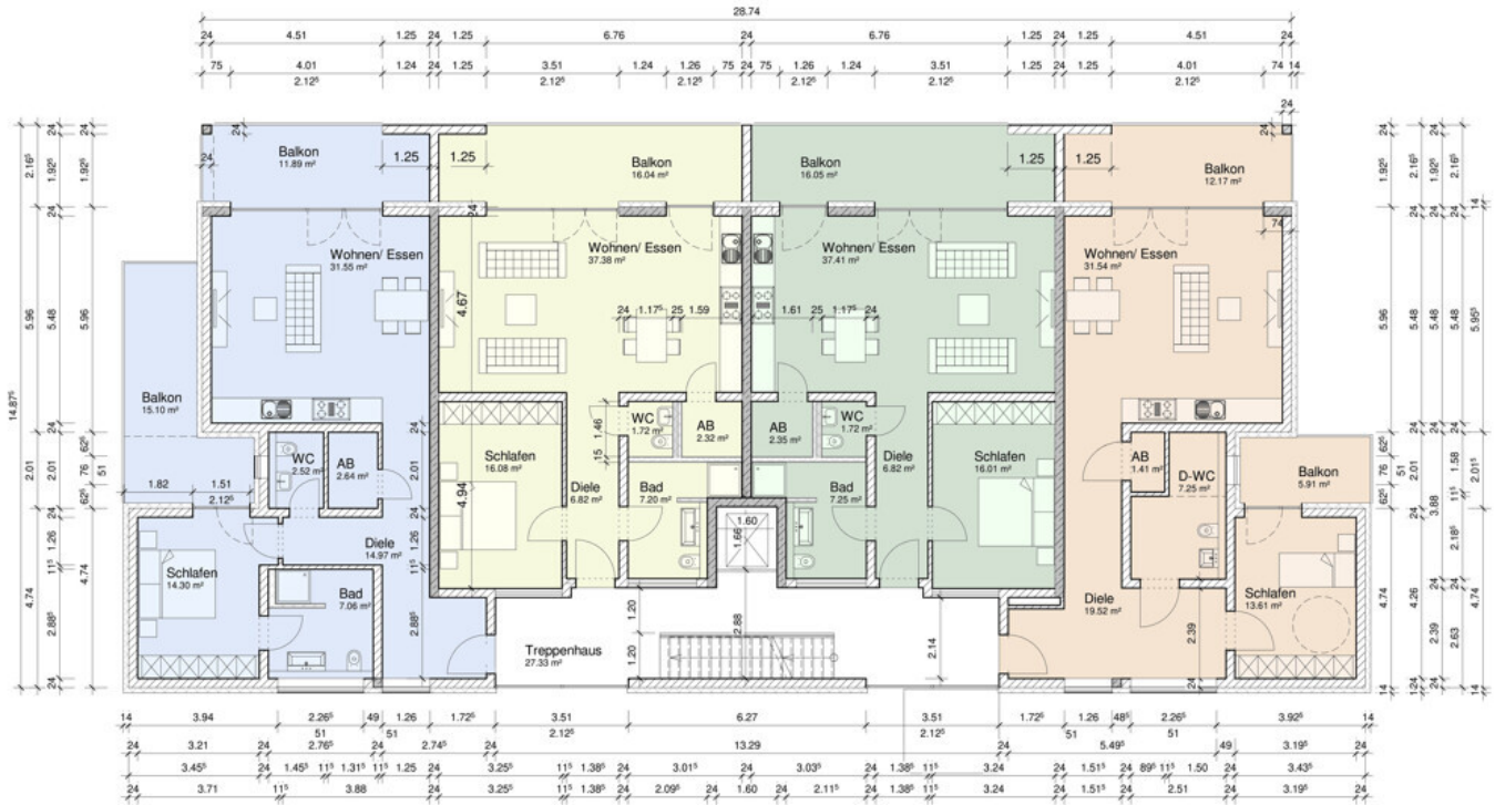
Luma Grundriss 1. Obergeschoss bemaßt
