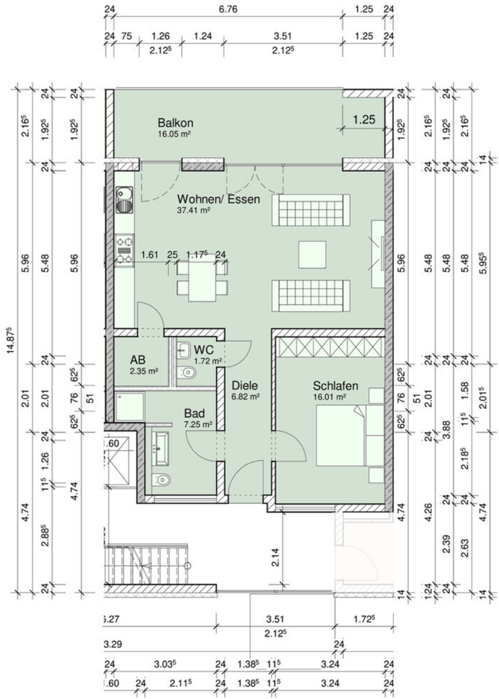
Luma Grundriss Wohnung 3 bemaßt
