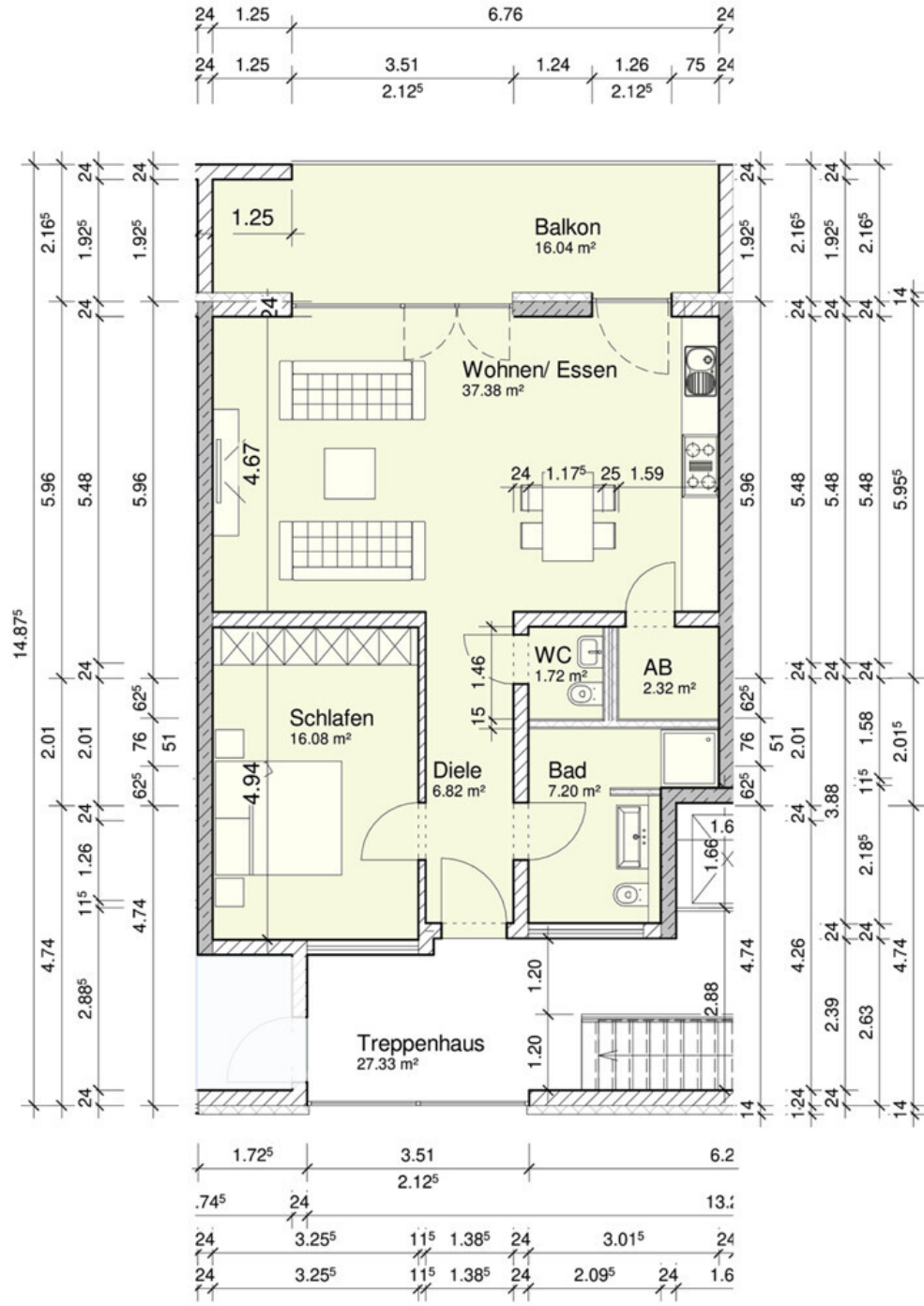
Luma Grundriss Wohnung 2 bemaßt
