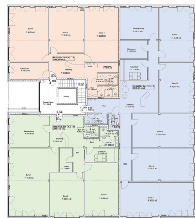
Gebäude 2_OG
